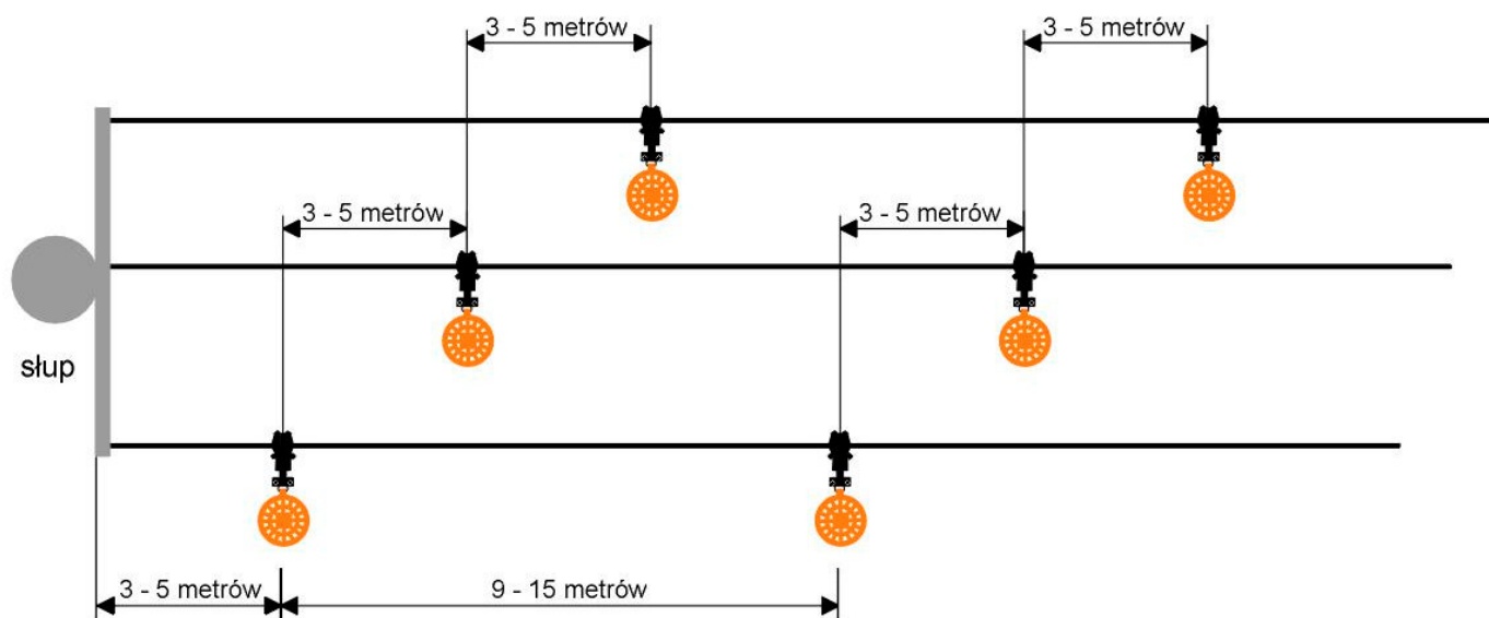
Rysunek 2. Zalecane rozmieszczenie odstraszaczy ptaków typu KS70
