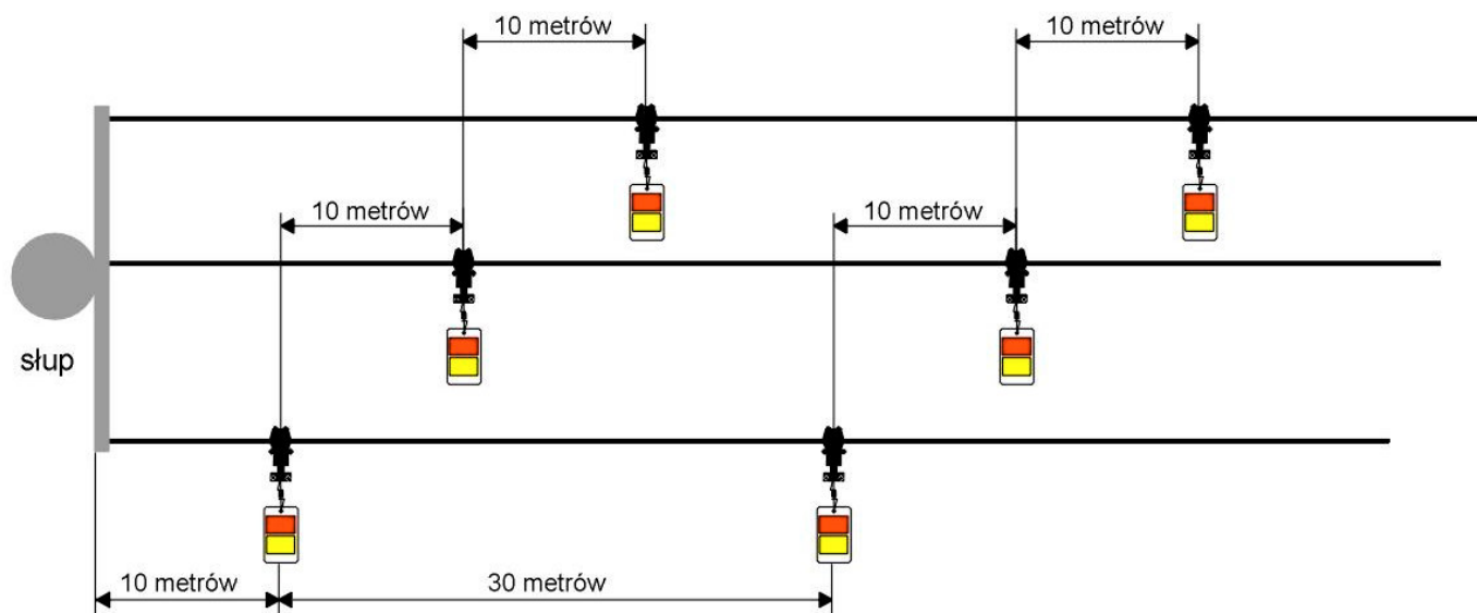
Rysunek 1. Zalecane rozmieszczenie odstraszaczy ptaków typu FireFly KS75
